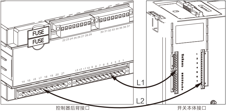
C1型控制器端子接线图
