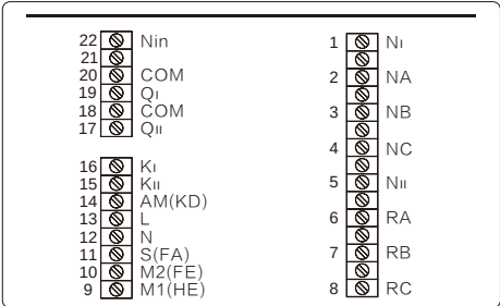
开关本体接口接线图 (XDQ1-800)
