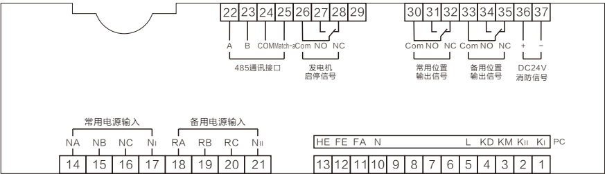
C1型控制器端子接线图
